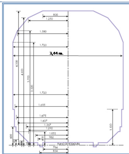
Gálbo de ancho ibérico (1.668 m.)
