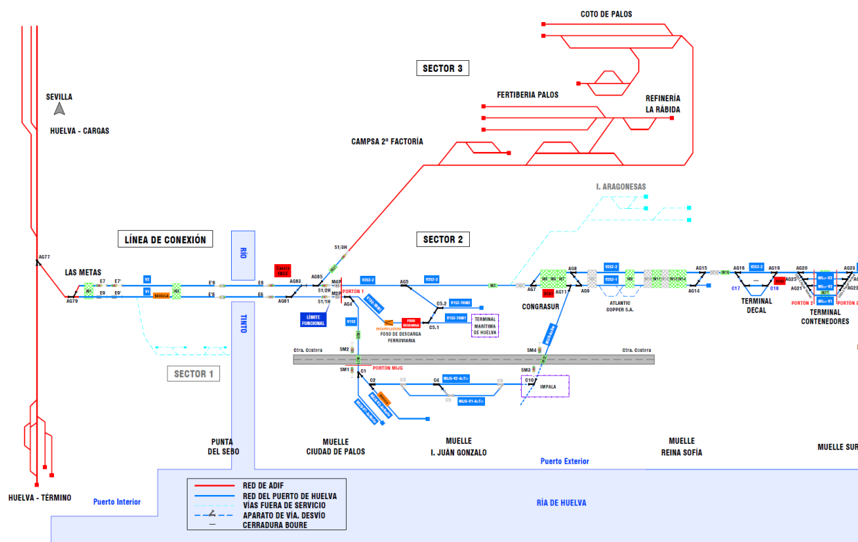
Esquema de vías de la RFAPH
